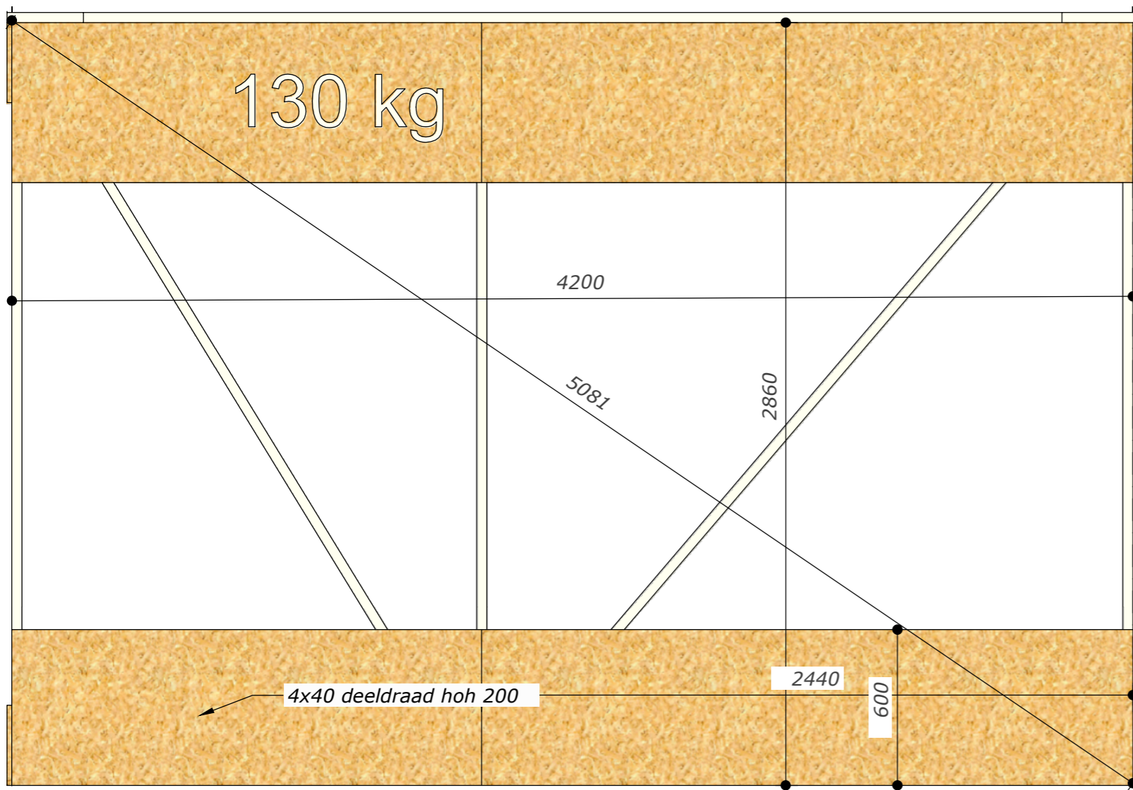
Bovenaanzicht 1:20
