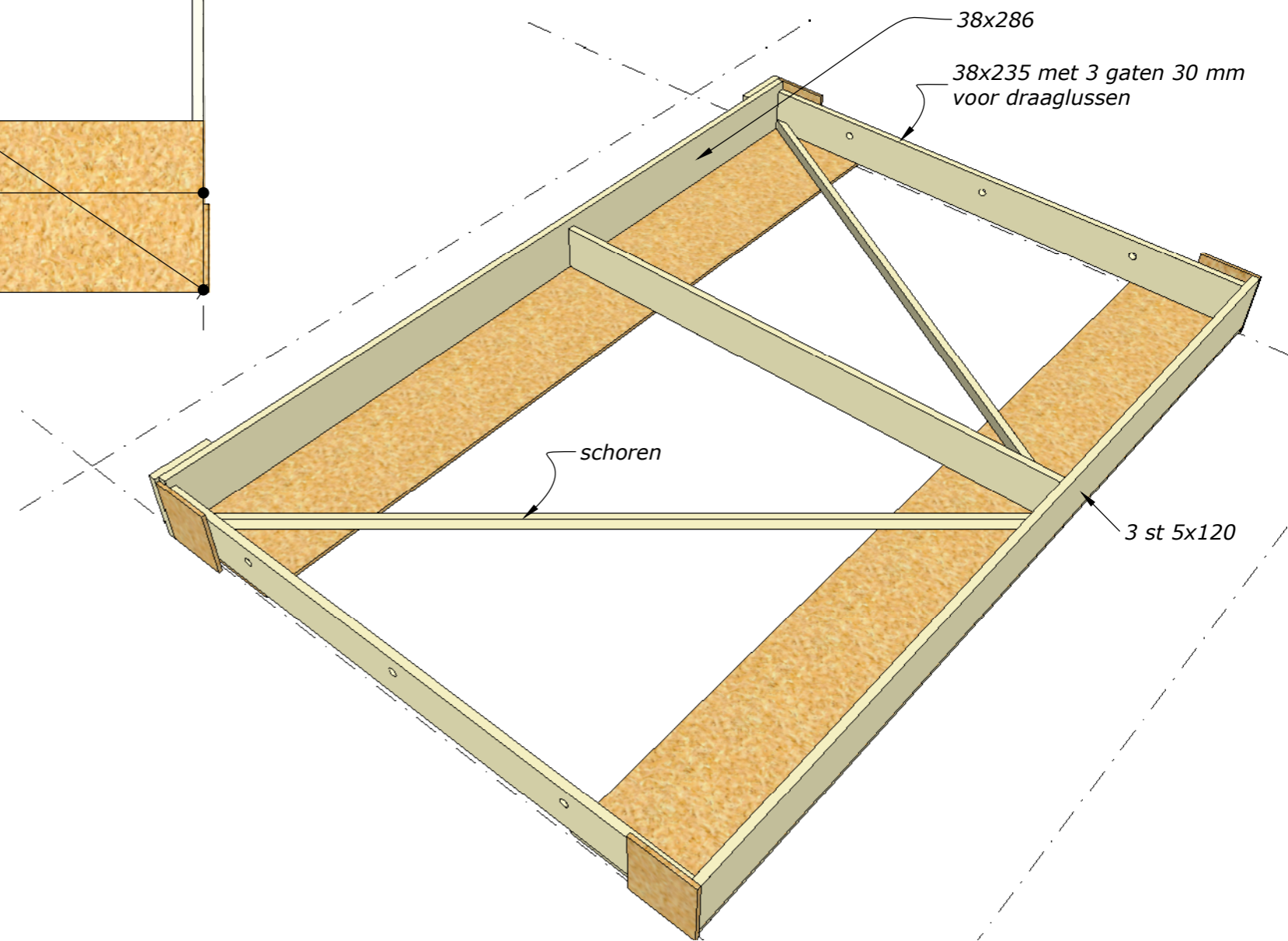
Perspectief onderkant
