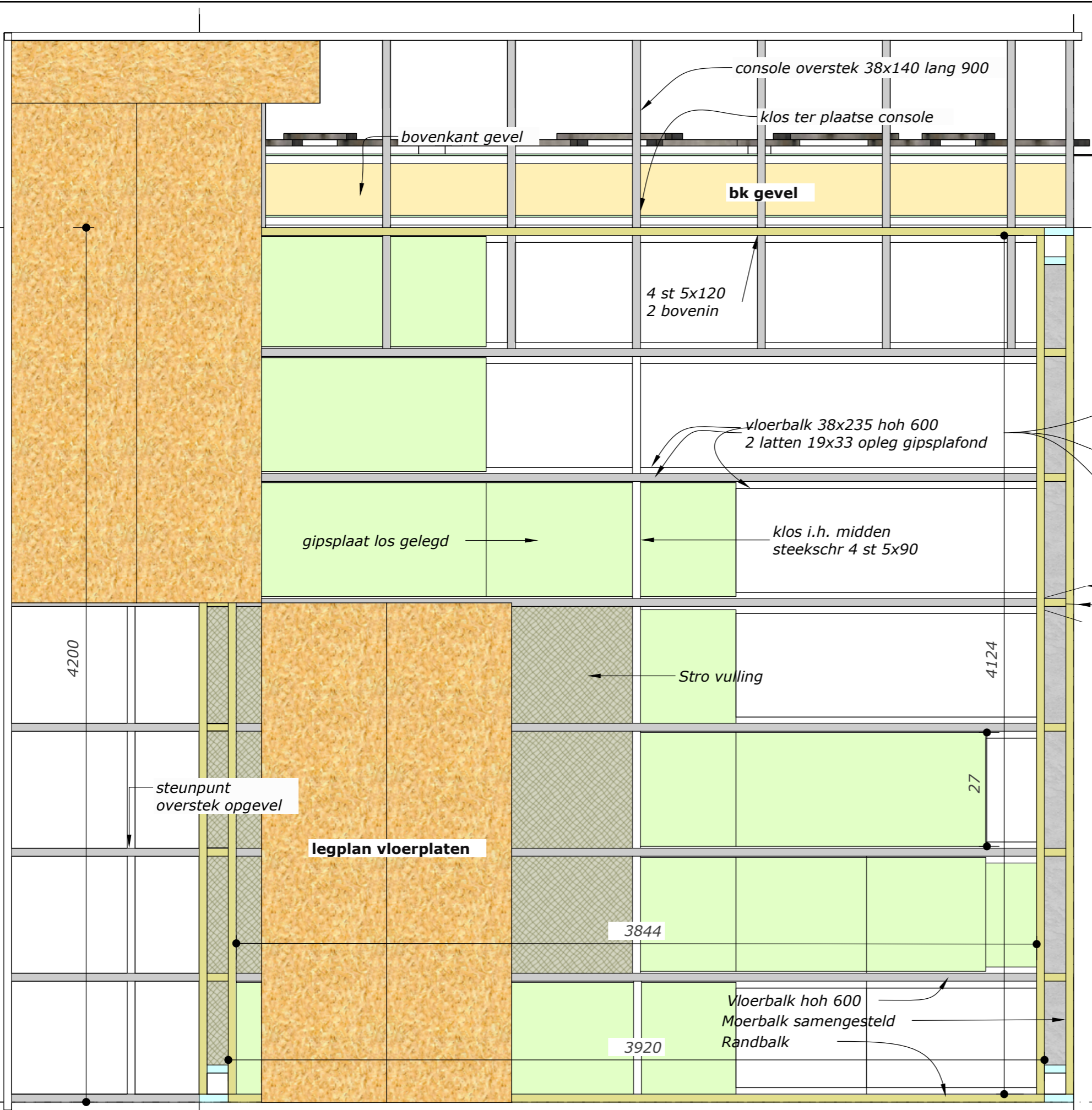
Verdiepingsvloer 1:20
