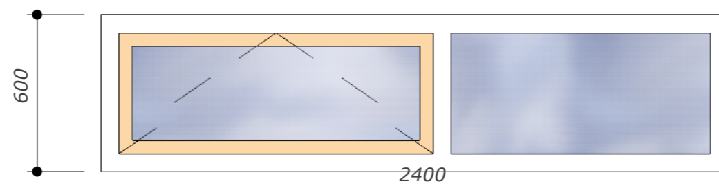
Raam hoog en boven aanrecht 2 st 1 naar binnen draaiend val raam
