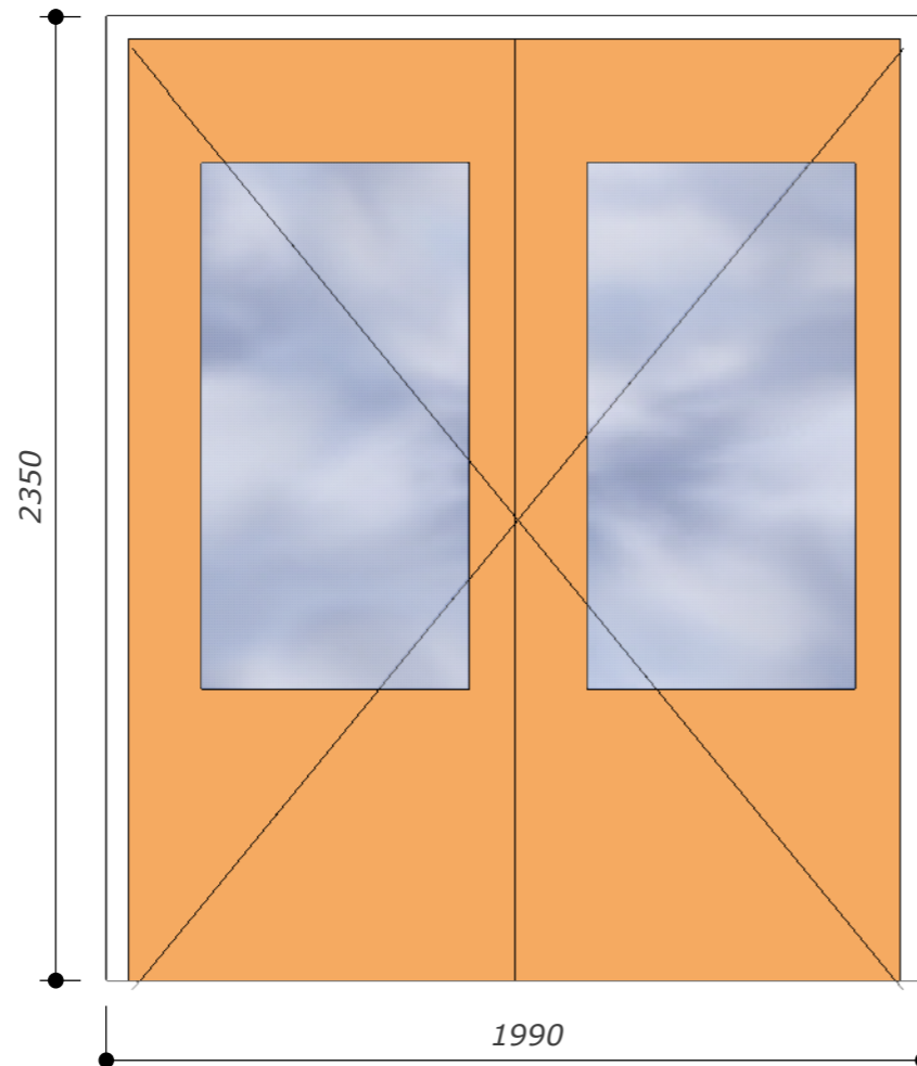
Dubbele deur naar buiten draaiend 2 st deurmaat 930 breed minimaal 2100 hoog
