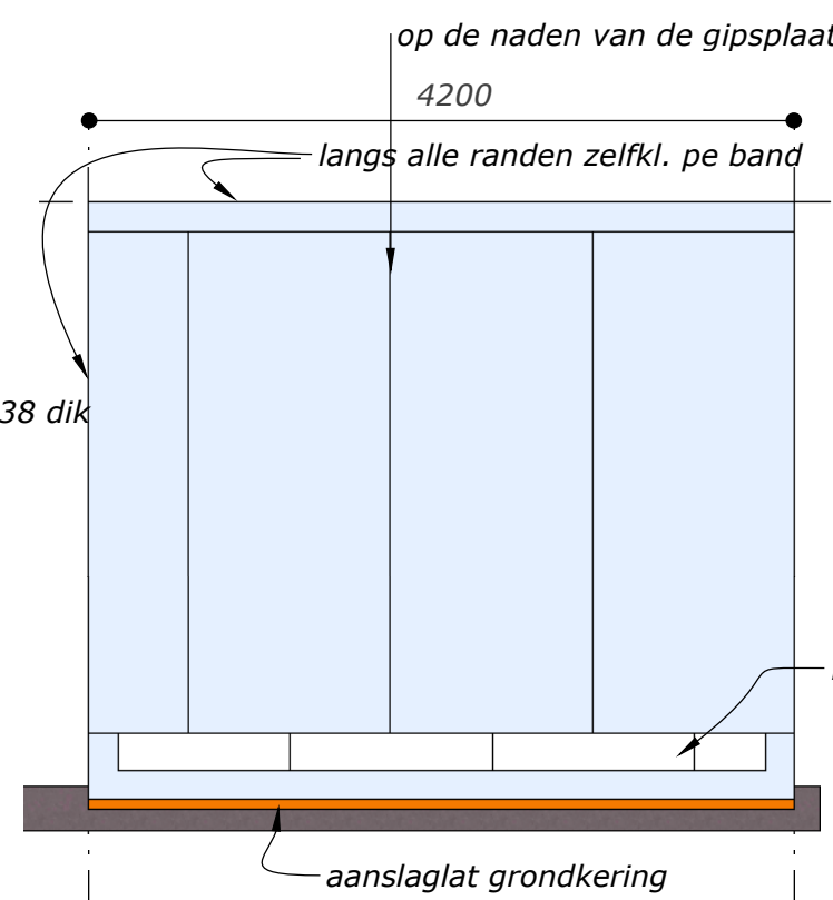
Stadium 4 gipsplaat 12,5 mm binnenafwerking
