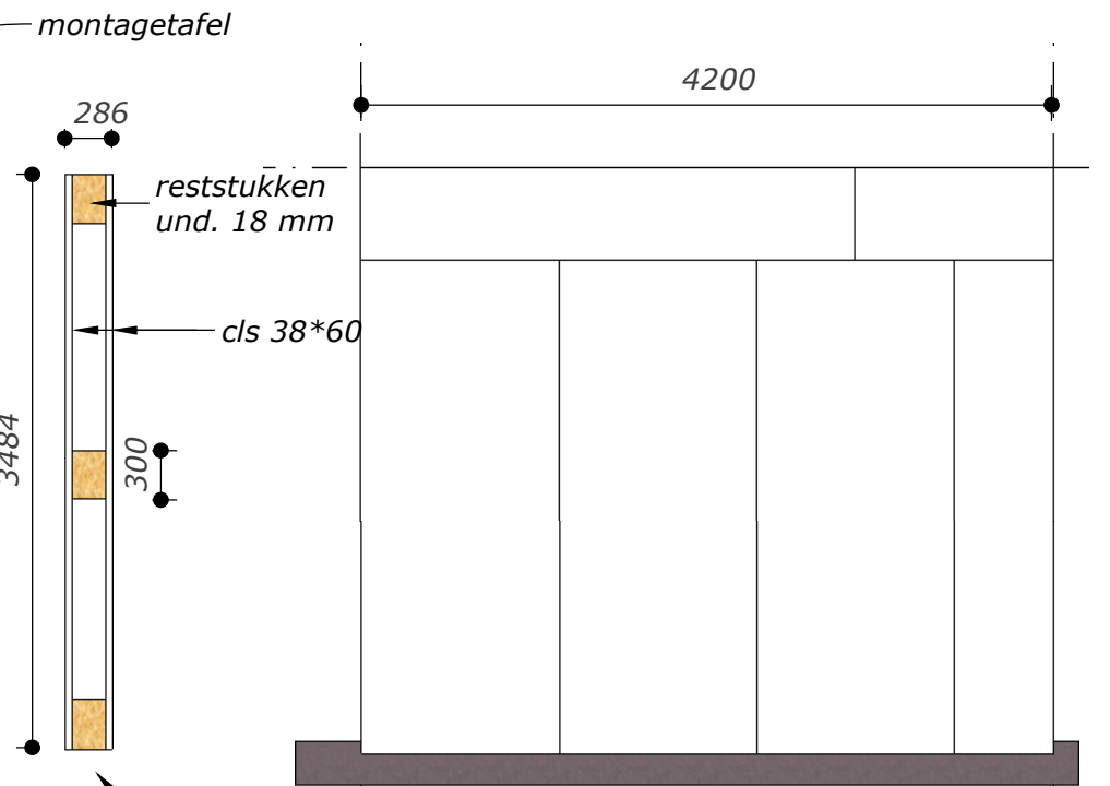
Stadium 2 gipsplaat tussenlaag grijs 12,5 mm
