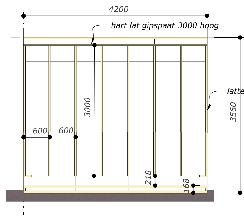
Stadium 3 Raamwerk voor leidingen
