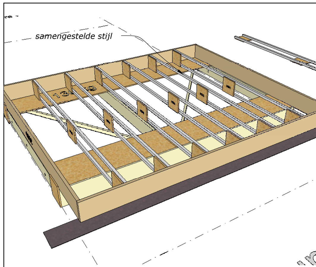
Perspectief vloer op montagetafel
