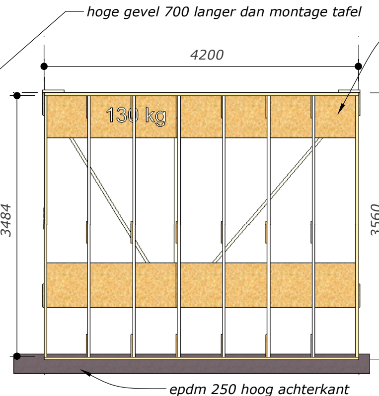
Stadium 1 Raamwerk 38x286 met samengestelde stijlen 38x286
